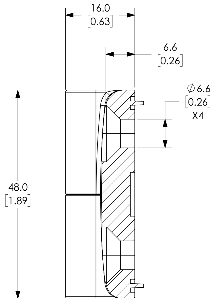
SECTION A-A
