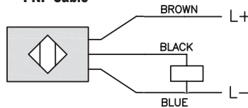
PNP Cable
