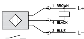
NPN Output
