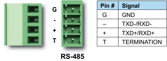
Port 4
