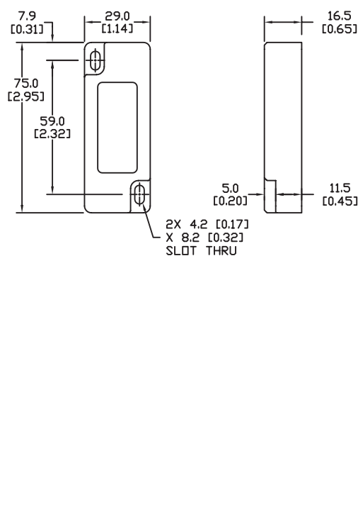
ACTUATOR
