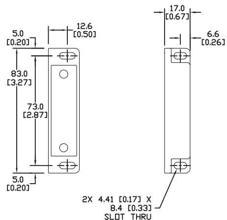
ACTUATOR
