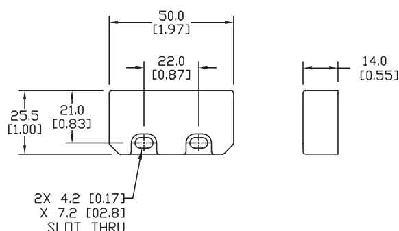
ACTUATOR
