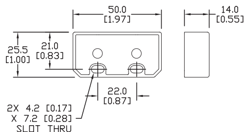
ACTUATOR
