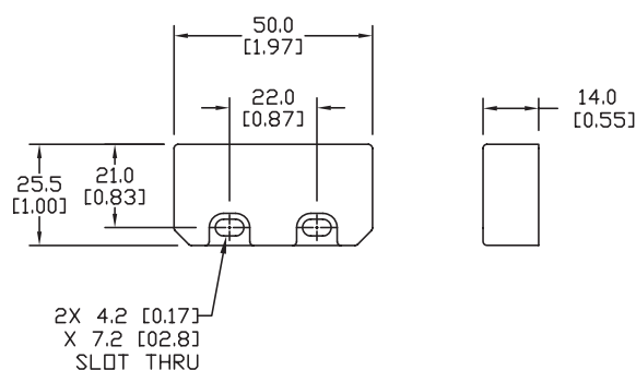
ACTUATOR
