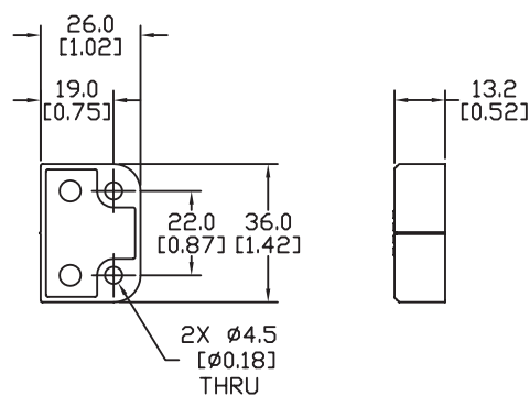
ACTUATOR
