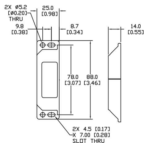
ACTUATOR
