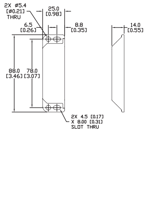
ACTUATOR
