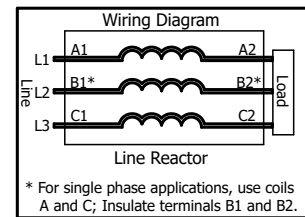
Wiring
