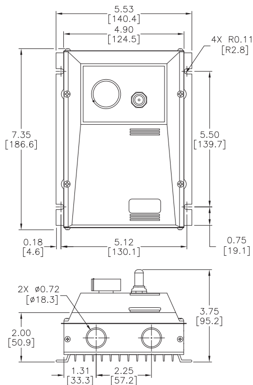
GSD5-240-10N4-x Dimensions
