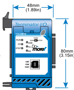
CPU Module
