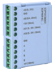
CFW320-IOAENC
