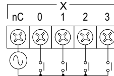
AC Input
