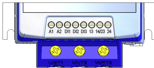
Figura 3.9 - Bornes de controle da SSW-07
