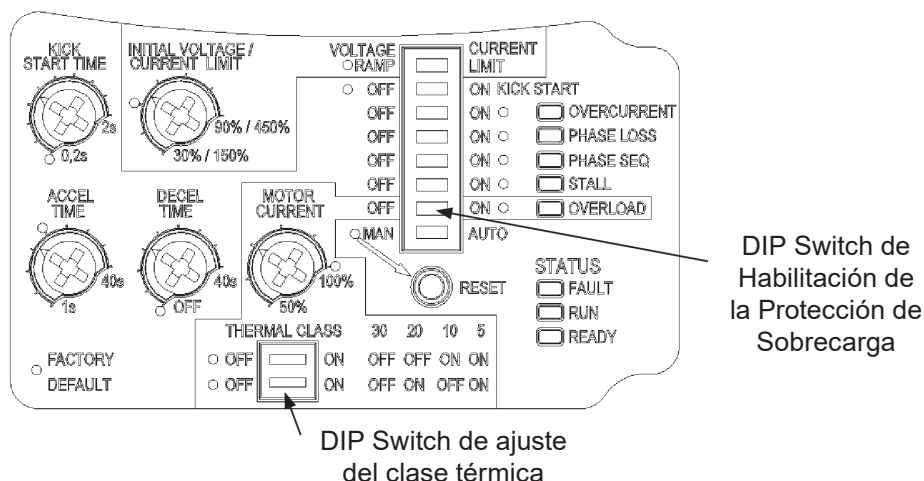
Figura 4.10 - Habilitación e ajuste de la protección de sobrecarga
