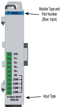
Analog Input Modules
