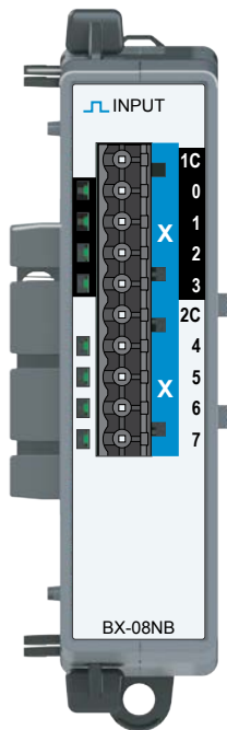
BX-08NB Input Module 8-pt, 12–24 VAC
