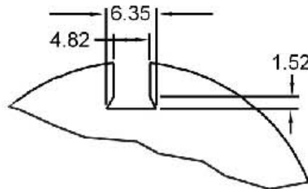
GROOVE DIMENSIONS
